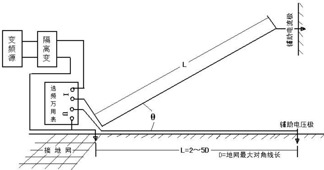
图 4-3 夹角法接线示意图
