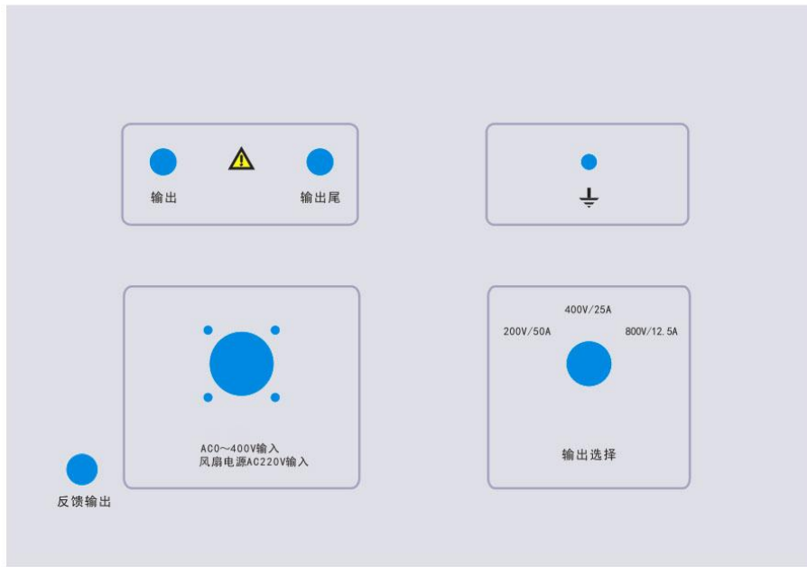
隔离变压器面板图
