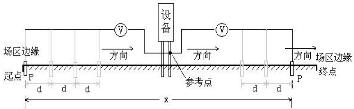
图 4-4 场区地表电位梯度分布测试示意图
