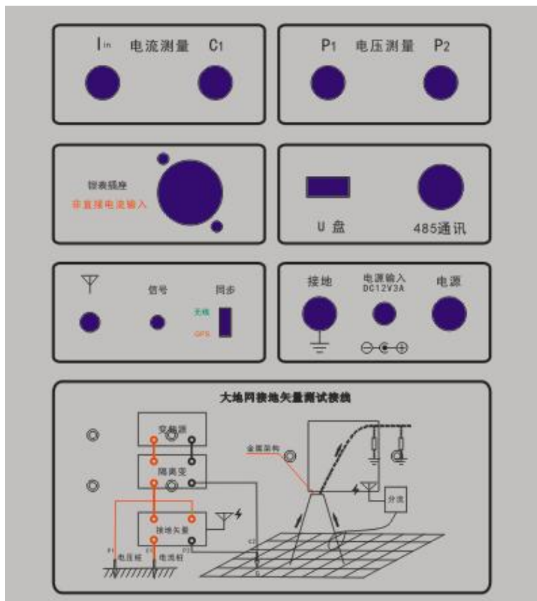
大地网接地矢量测试装置面板图
