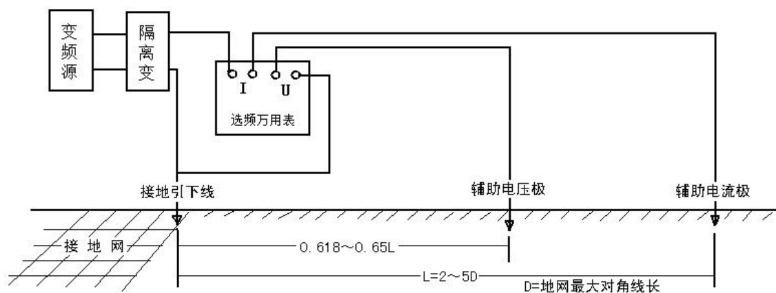
图 4-2 直线法接线示意图
