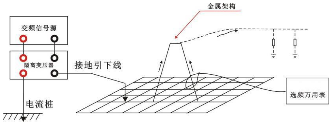
图 4-7 分流有效值测试接线示意图
