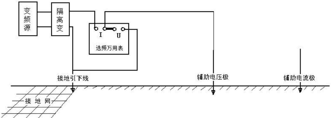
图 4-9 电压桩电阻测试示意图
