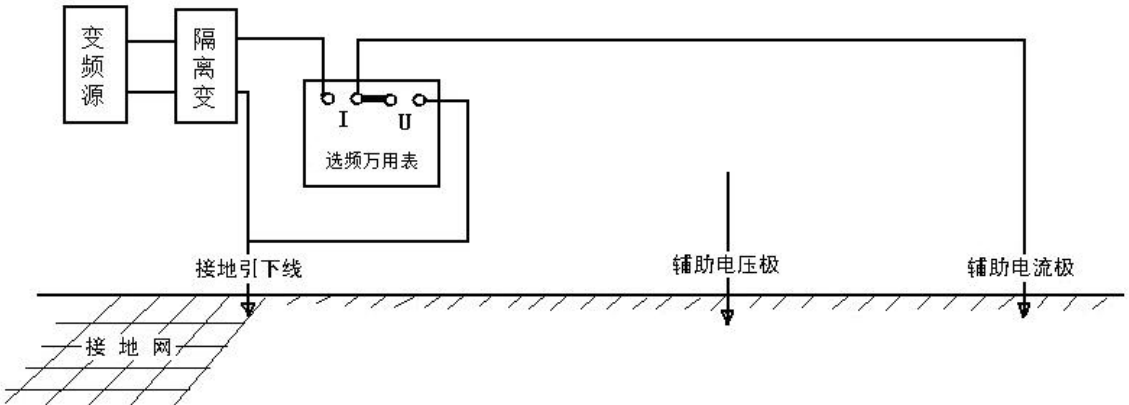
图 4-8 电流桩电阻测试示意图
