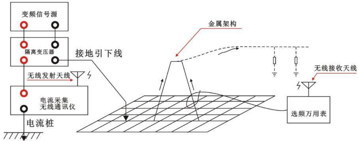
图 4-6 分流向量测试接线示意图
