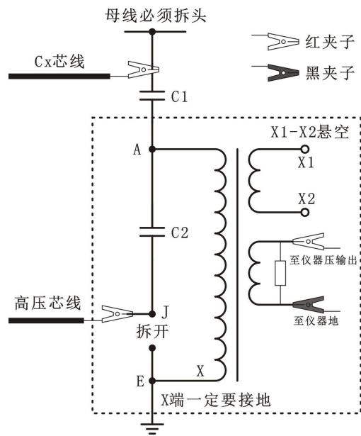
图 5-6 110kV CVT 测量 C1 和 C2 参考接线
