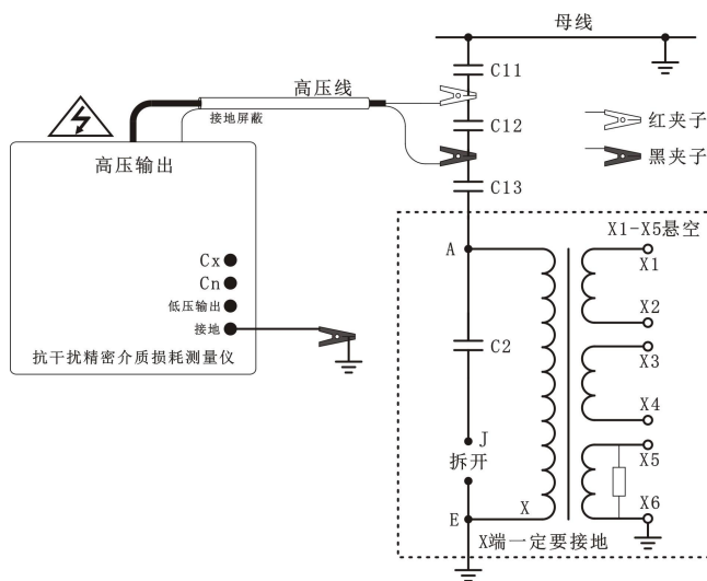
图 5-1 500kV CVT 测量 C11 参考接线
