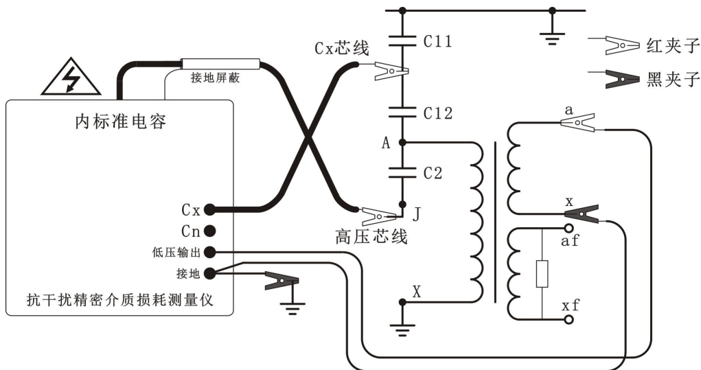
图 4-10 CVT 自激法参考接线图
