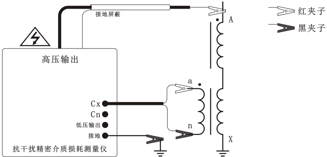
图 4-11 电磁式 PT 变比参考接线图
