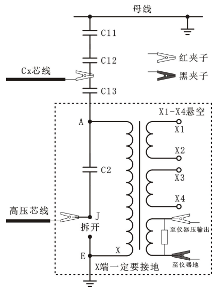
图 5-3 500kV CVT 测量 C13 和 C2 参考接线
