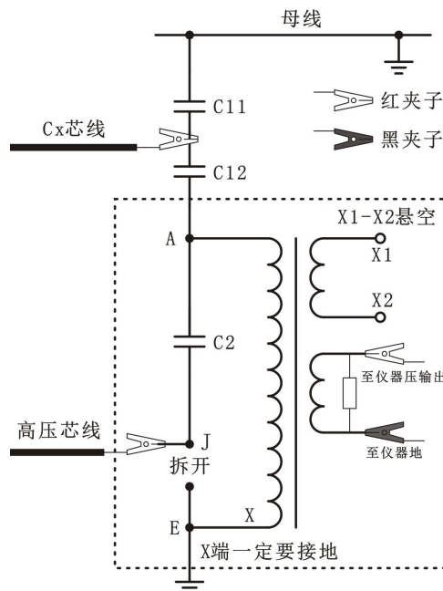
图 5-5 220kV CVT 测量 C12 和 C2 参考接线
