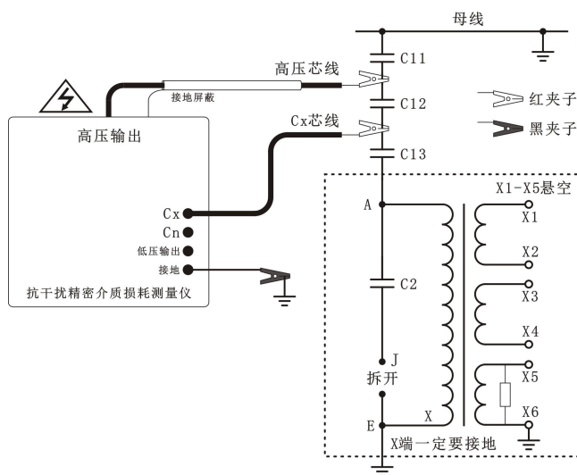
图 5-2 500kV CVT 测量 C12 参考接线
