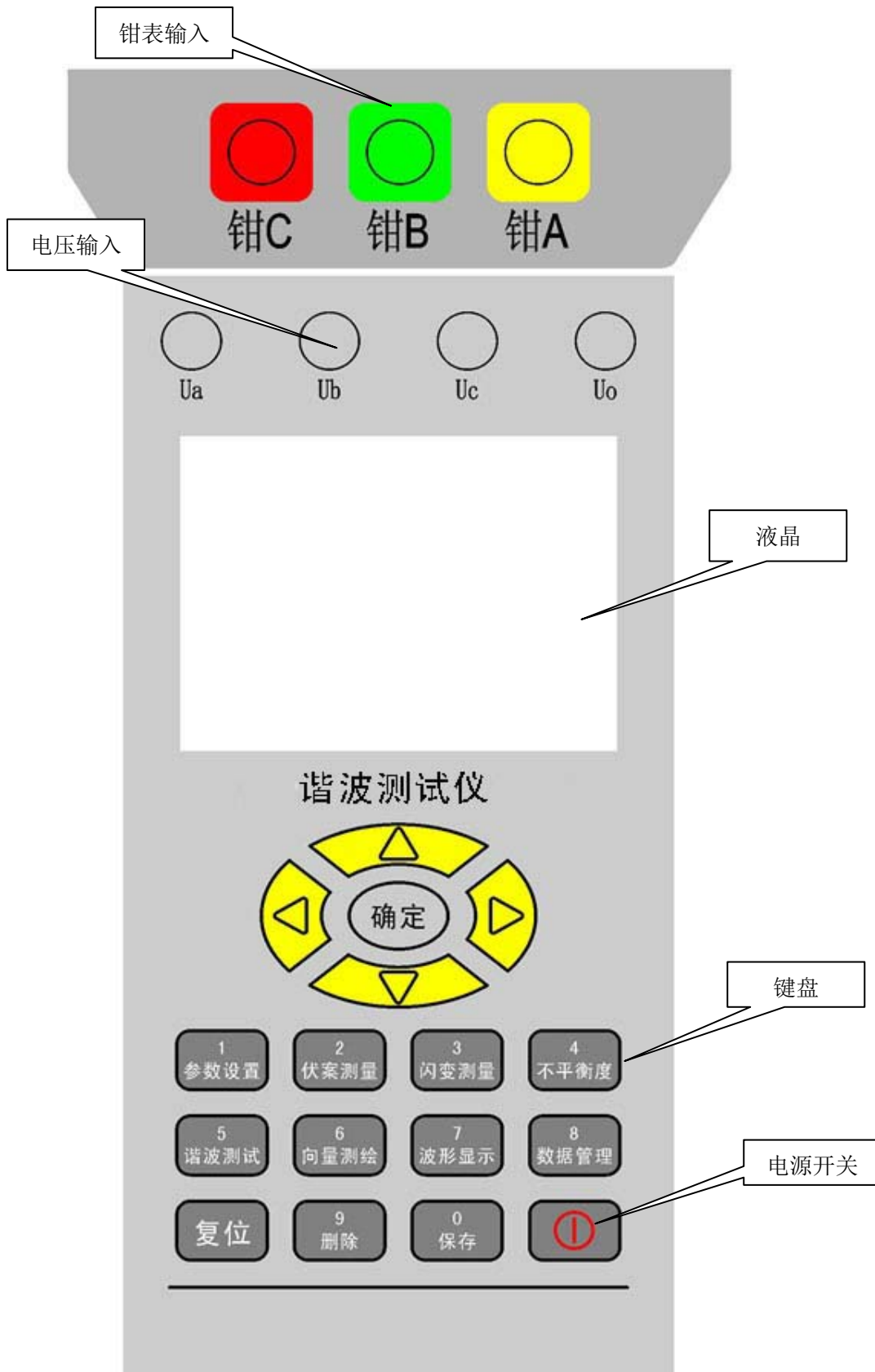
图1 面板布置图
