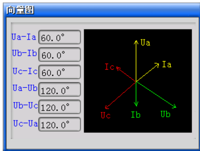
图8 向量图
