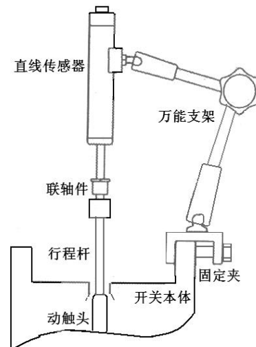
油开关直线测速安装示意图
