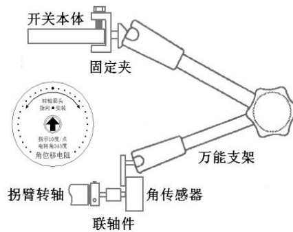
角度测速安装示意图
