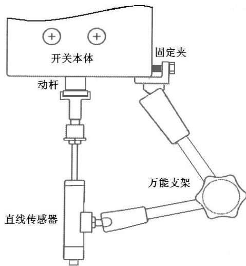
真空开关直线测速安装示意图
