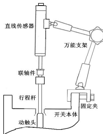
油开关直线测速安装示意图
