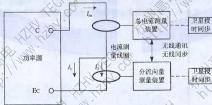
图 A-1 主从模式工作原理
