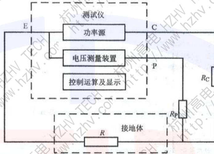
图中：C——电流极； P——电压极； E——电压、电流公共极； R——（被测接地体）的等效接地电阻； R C ——电流极等效辅助接地电阻； R P ——电压极等效辅助接地电阻。
