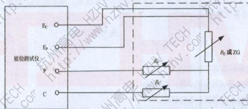
图中： E_p ——电压（电位）极端子； E_c ——电流极端子。
