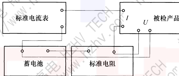
图 1 蓄电池内阻测试仪电阻器校验接线
