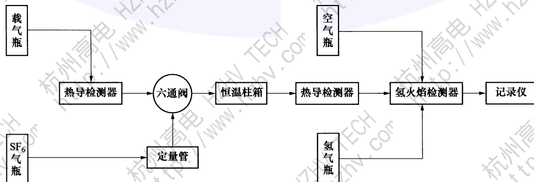
图 1 空气、四氟化碳、六氟乙烷和八氟丙烷测定装置示意图
