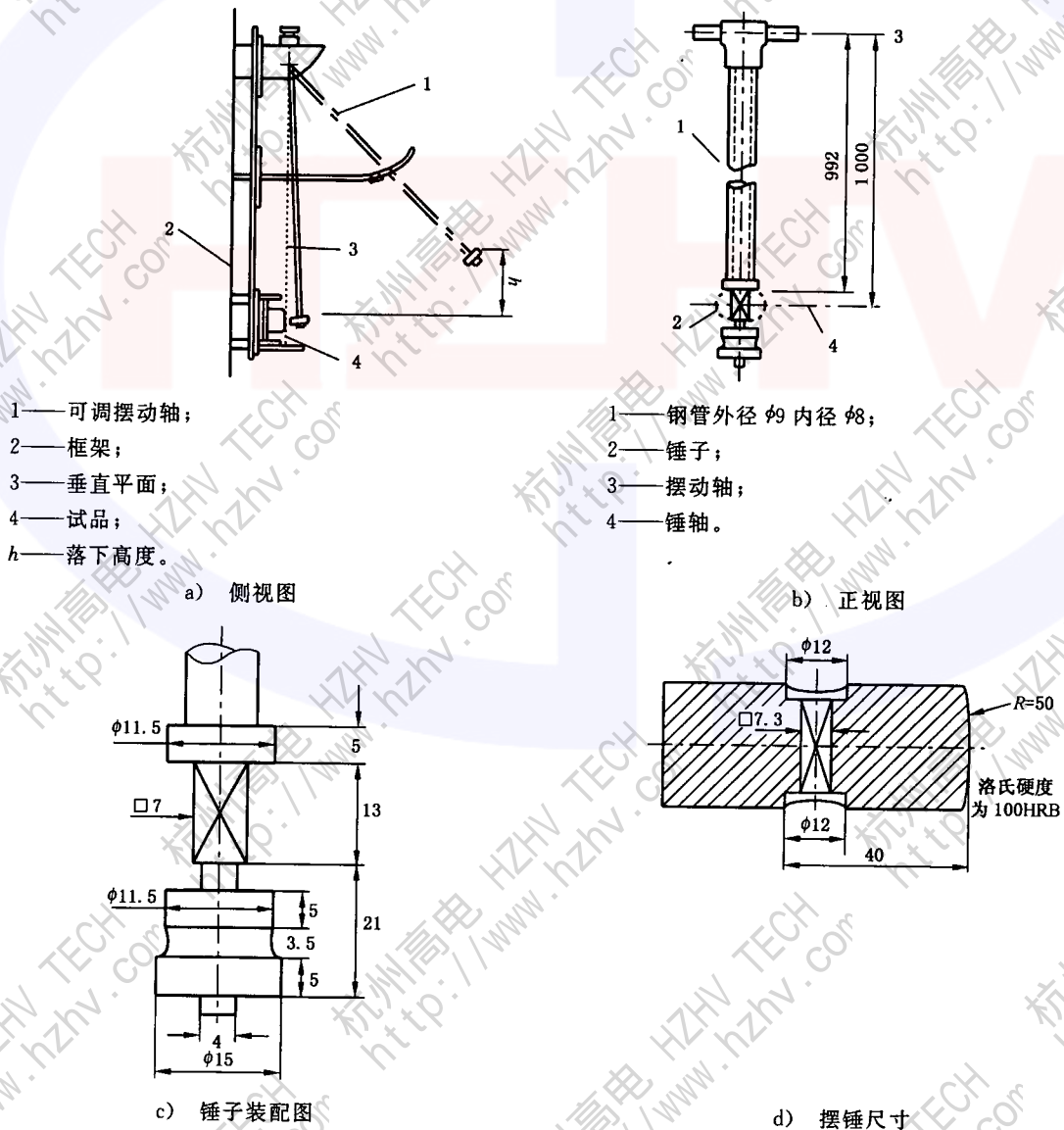
图 D.1 冲击试验摆锤法
