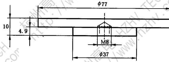
a) 2个黄铜电极
