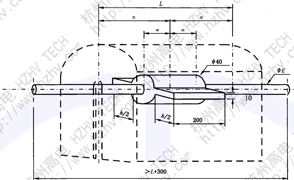
图 F.3 棒形绝缘子遮蔽罩的电极
