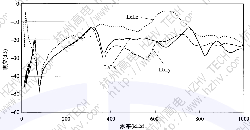
图 I.5 SF9-3150/110 变压器低压绕组变形时的幅频响应曲线
