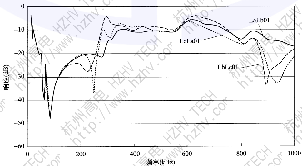
图 I.7 SFZ-3150/110 (H) 变压器低压绕组变形时的幅频响应曲线
